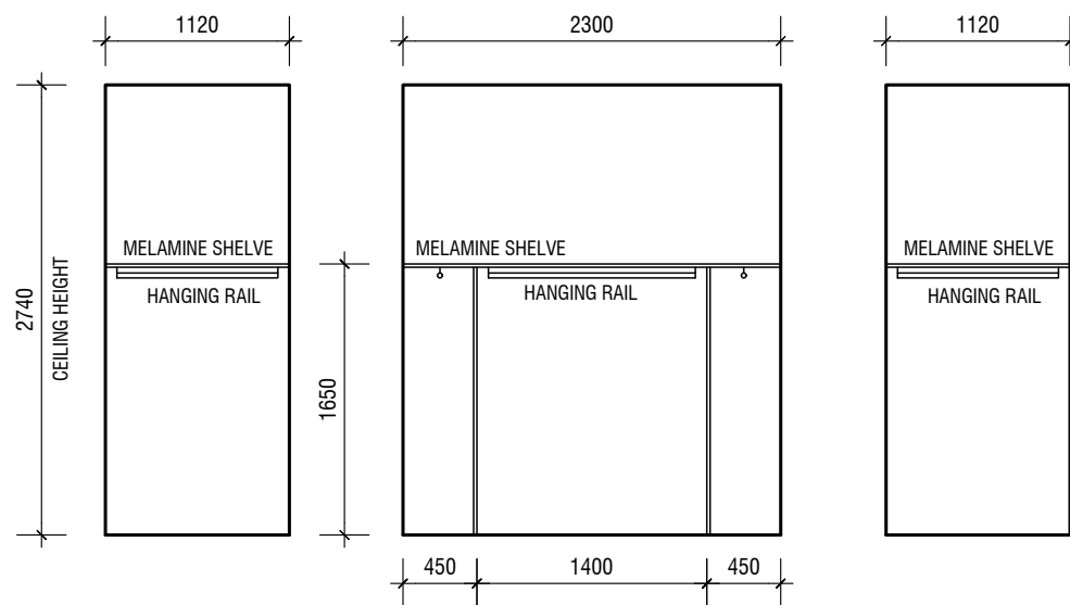
ELEVATION A
