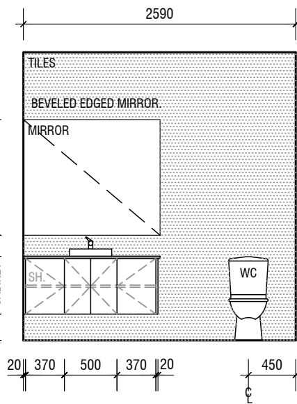
ELEVATION B
