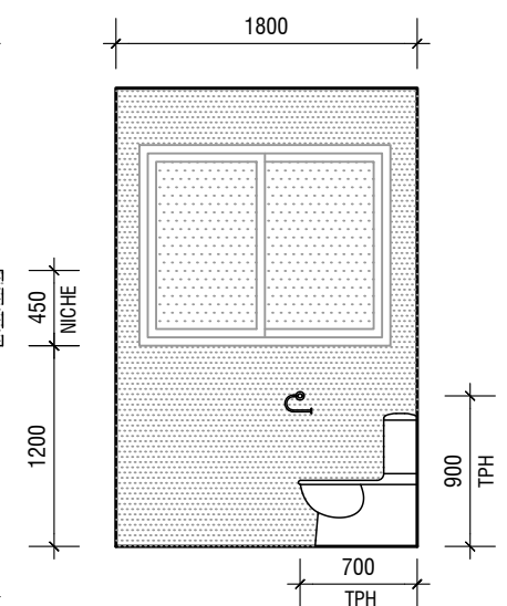
ELEVATION E
