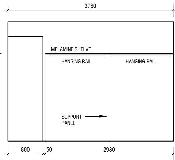
ELEVATION B
