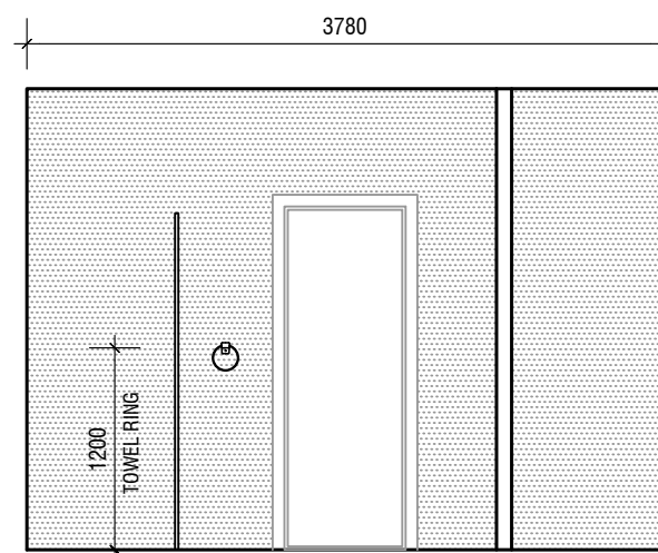
ELEVATION B
