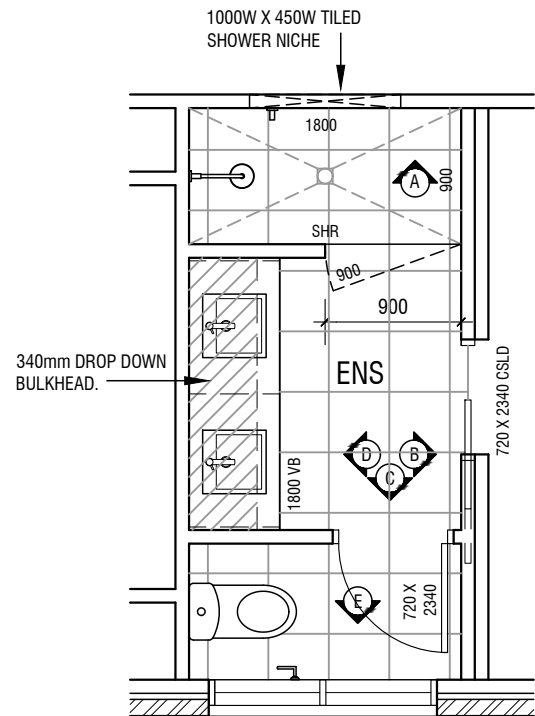
ENSUITE PLAN
