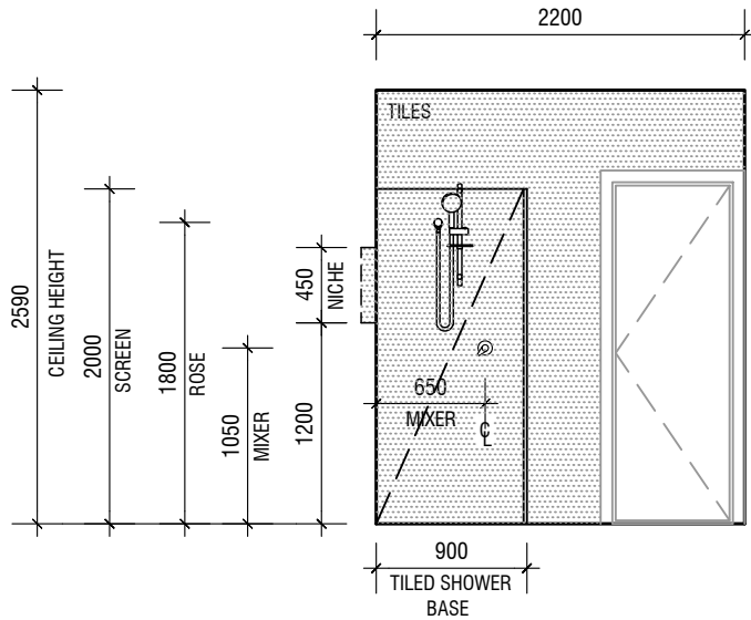
ELEVATION A
