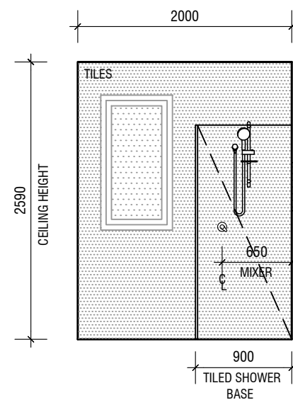
ELEVATION A
