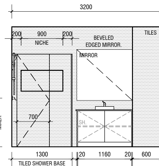
ELEVATION B
