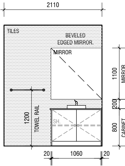
ELEVATION B
