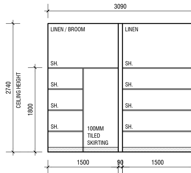
ELEVATION A
