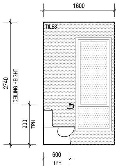
ELEVATION A
