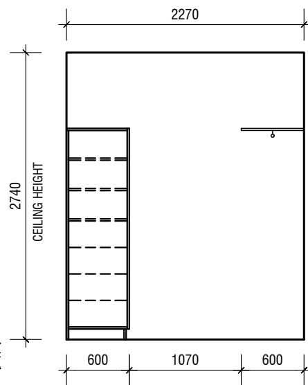
ELEVATION A
