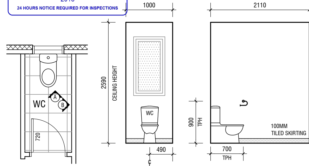
WC PLAN
