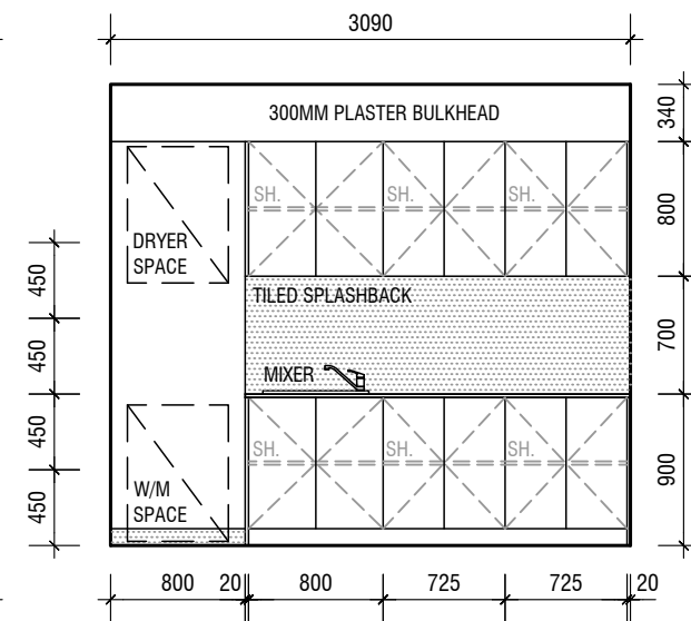
ELEVATION B
